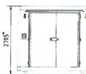
DOOR ELEVATION
